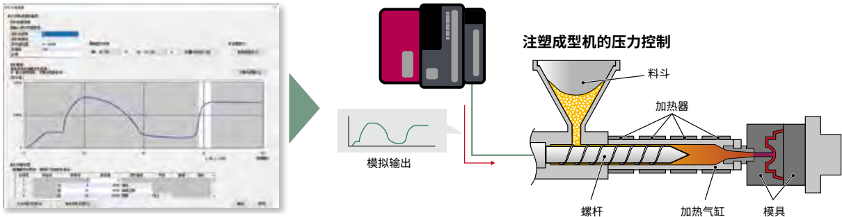
工程设计软件GX Works3的波形输出设置画面
