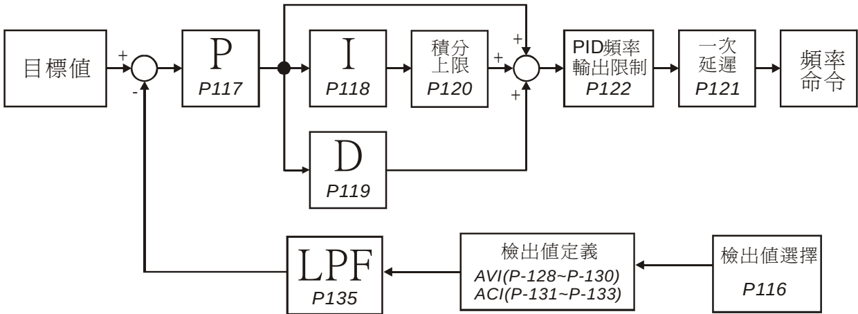
PID控制方塊圖
