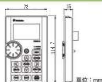
PU301C 尺寸圖
