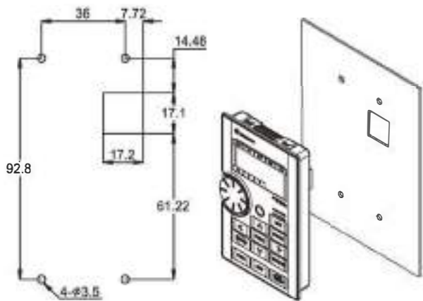
盤面安裝開孔尺寸圖：
