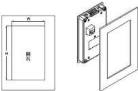
卡扣安裝開孔尺寸圖：
