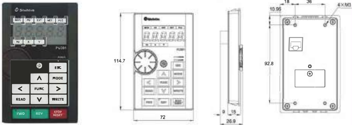
外觀及尺寸圖：
