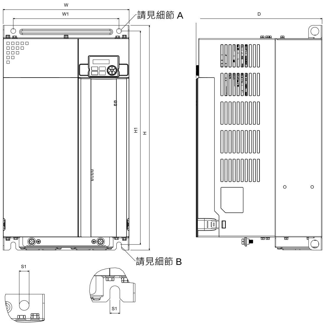
細節 A (安裝孔) 細節 B (安裝孔)
